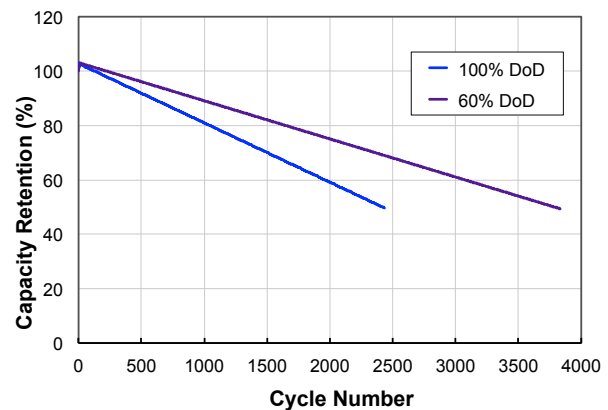
電池循環壽命
