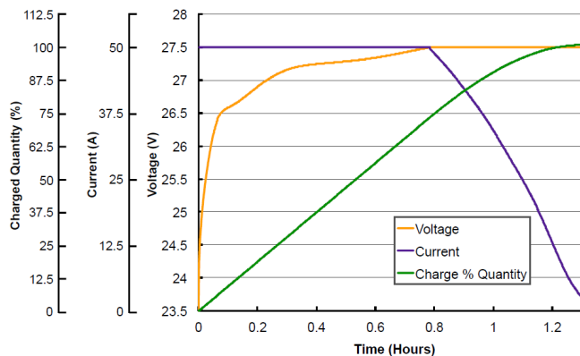
電池充電曲線 (50A, 1C)
